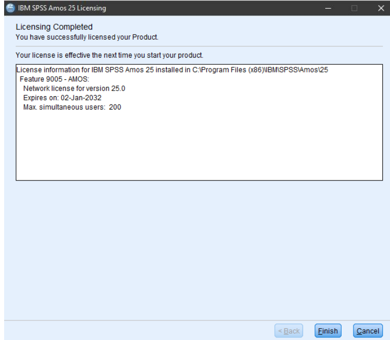
Şekil 15 Lisanslama İşlemleri
