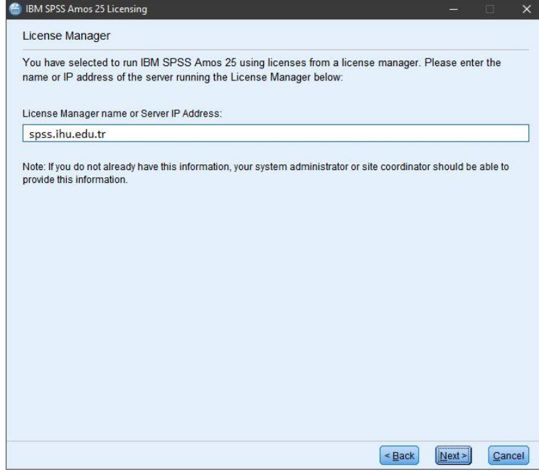
Şekil 14 Lisanslama İşlemleri
