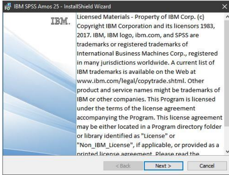
Şekil 1 Kurulumu Başlamak
