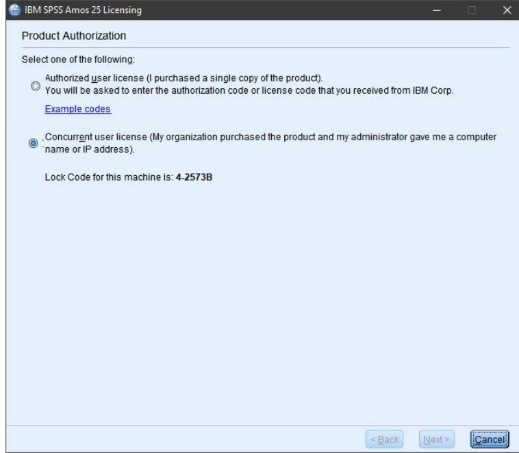
Şekil 13 Lisanslama İşlemleri
