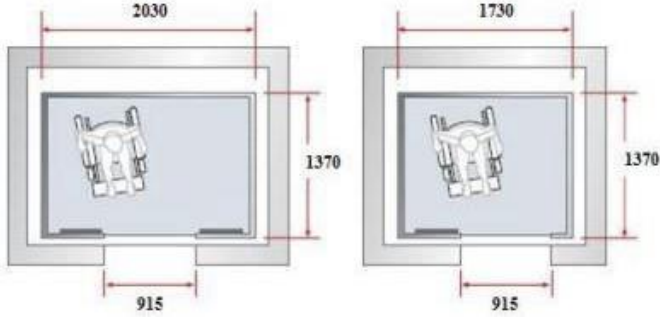
Şekil 10. Asansör kabini min. ölçüleri
