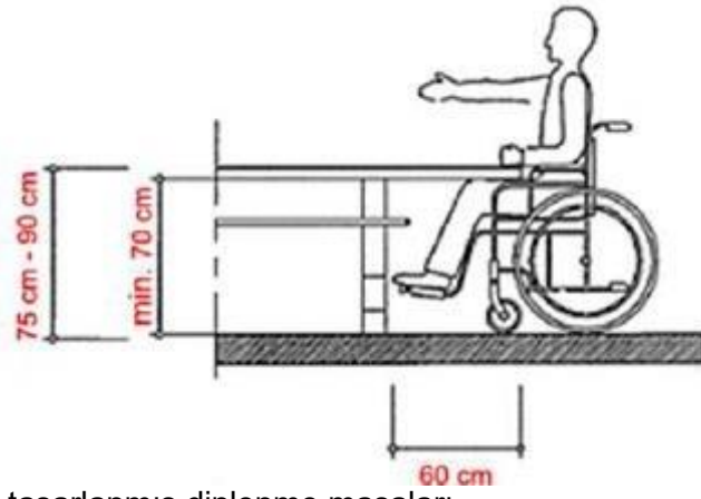
Şekil 17. Engelliler için tasarlanmış dinlenme masaları
