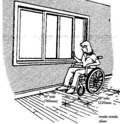
Şekil 8. Tekerlekli sandalyeli öğrencinin pencereye erişimi
