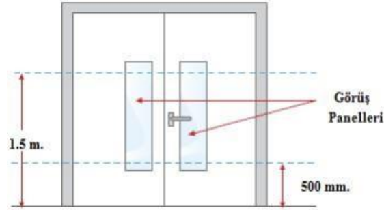
Şekil 7. Cam görüş panelleri yerleştirilmiş kapı
