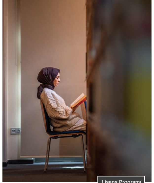
Lisans Programı
