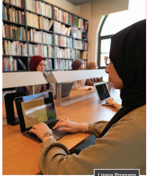
Lisans Programı
